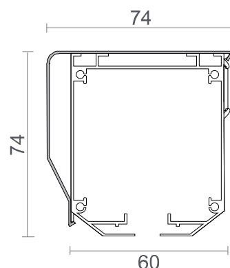
przekrój kasety z uchwytem wymiary podane są w mm
